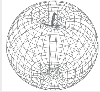
Şekil 4.2 Üç boyutlu elma çizimi
